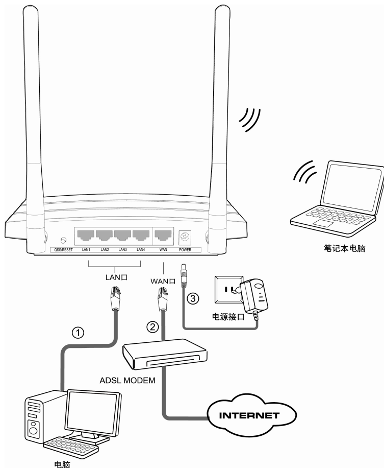
图 4-1 TL-WDR1100 硬件安装示意图
