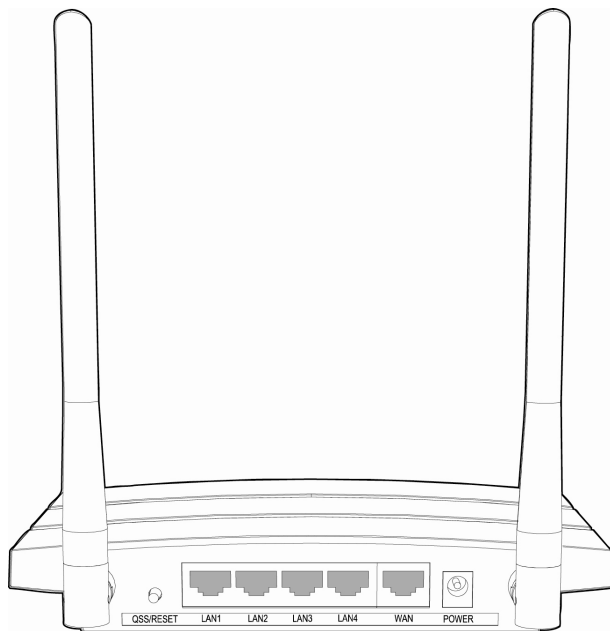
图 3-2 TL-WDR1100 后面板示意图
